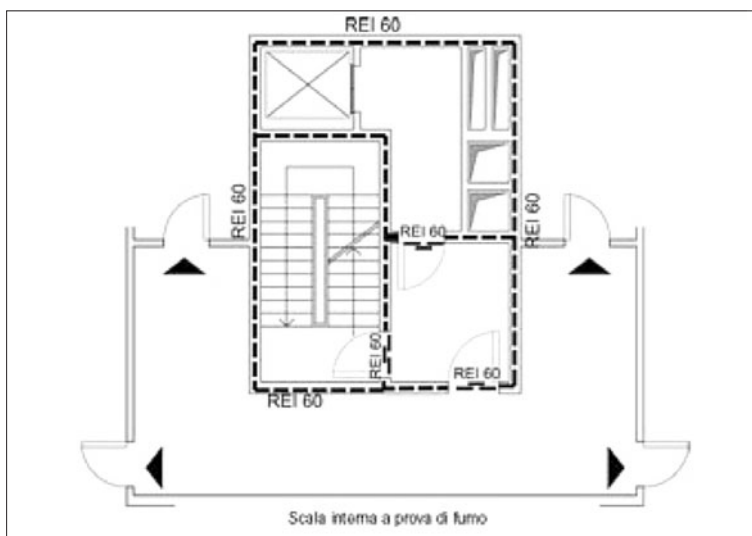
Scala a prova di fumo interna
