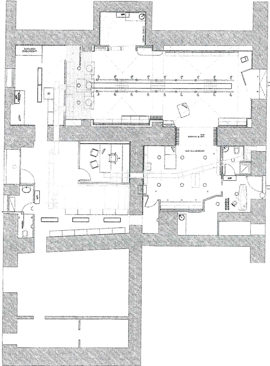
PIANTA LAYOUT FARMACIA "CIRILLO" scala 1:100
